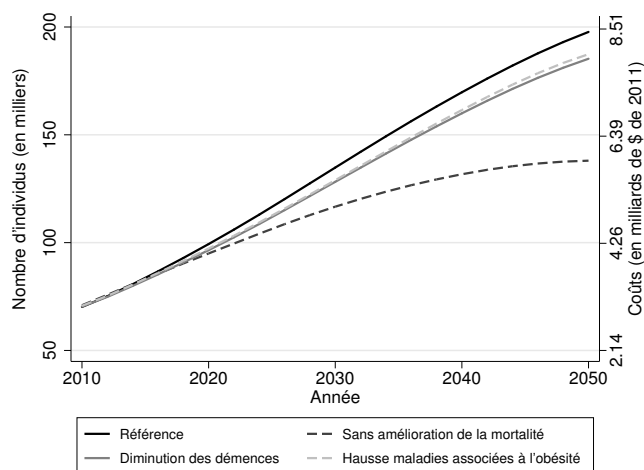
Figure 4 – Nombre d'individus en institution (en milliers, axe de gauche) et coût total (en milliards de dollars de 2011, axe de droite) de l'institutionnalisation. Les résultats sont présentés pour les 4 scénarios.
