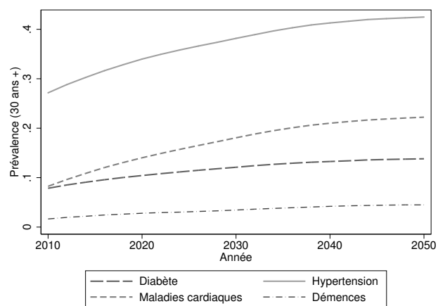
Figure 2 – Prévalence des maladies de 2010 à 2050. Source : Calcul des auteurs à partir de COMPAS.
