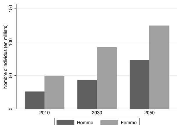
Figure 3 – Nombre d’individus (en milliers) en institution en 2010, 2030 et 2050, hommes et femmes séparément. Source : Calcul des auteurs à partir de COMPAS.
